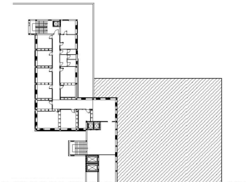
PIANO SECONDO
